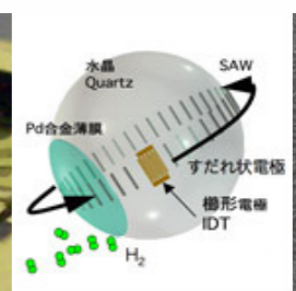
ボール SAW 水素ガスセンサの構造と原理
